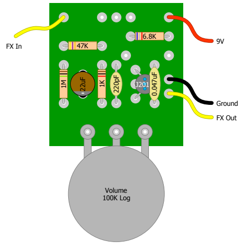
JFET Boost
